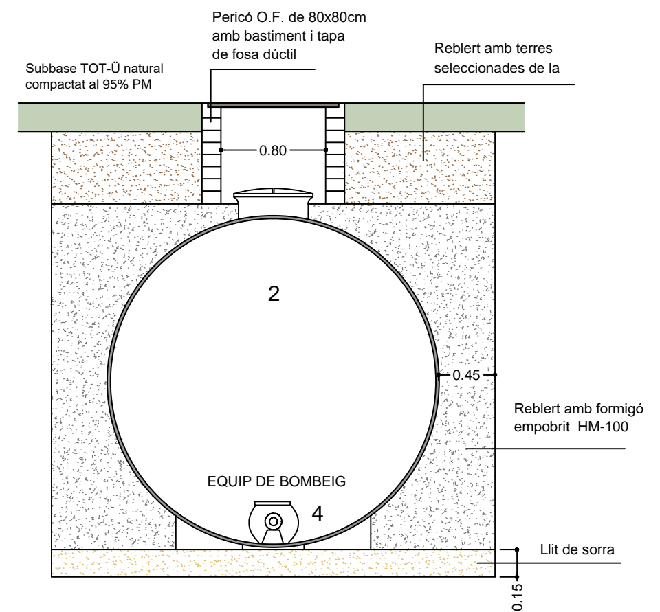
SECCIÓ TRANSVERSAL
